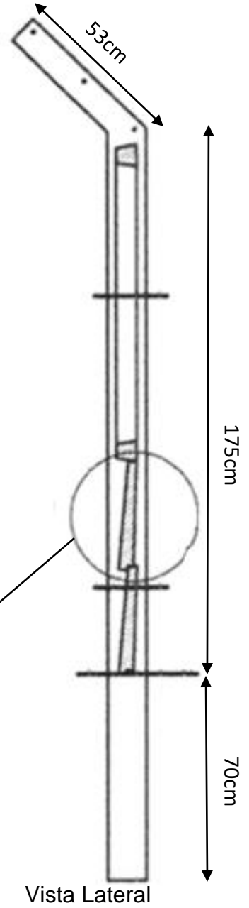
MURO CON CODO CALADO 1.75m
