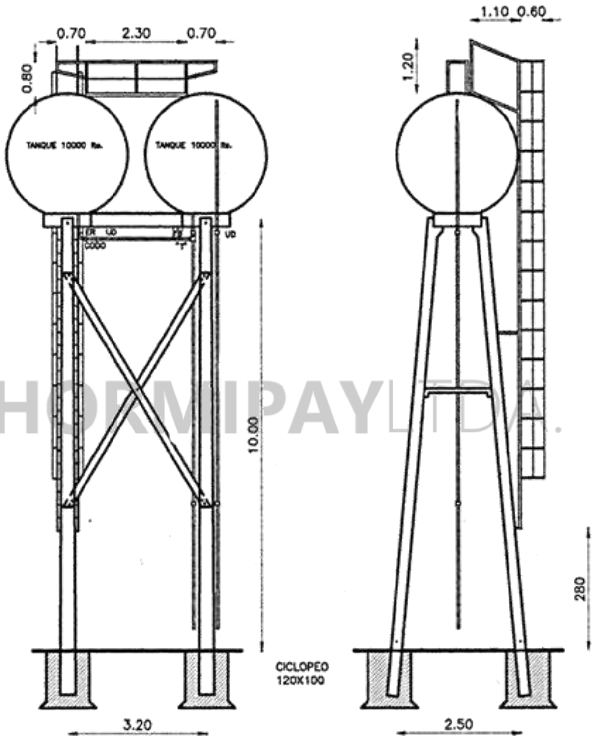
ALZADO FRENTE
