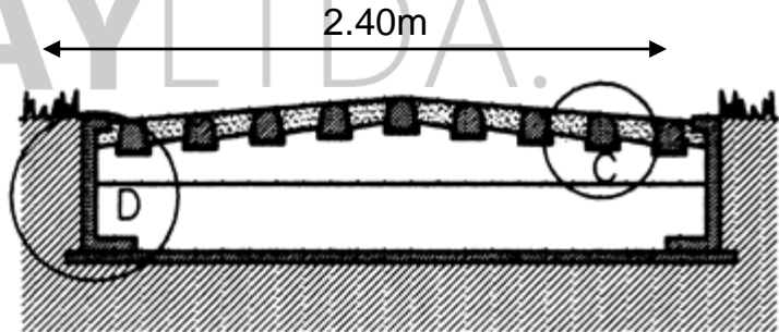
CORTE B-B
